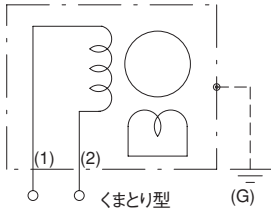
結線図
