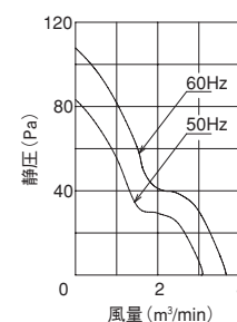
風量～静圧特性曲線
