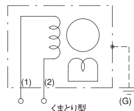
結線図
