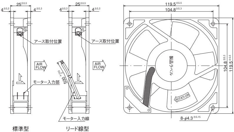
外形図
