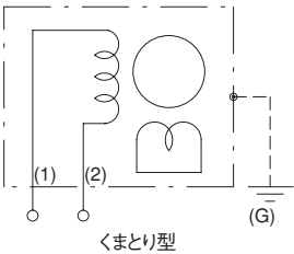
結線図
